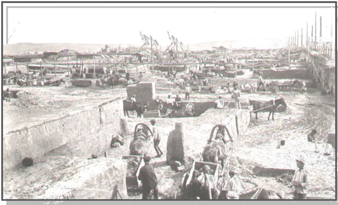
Строительство доменной печи Кузнецкого металлургического комбината. 1930 г.
